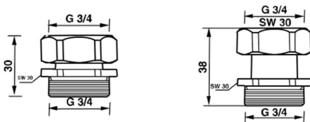
1 6220 71 Šroubení 3/4 s kónusem, s převlečnou maticí, napojení na potrubí 3/4 s plochým těsněním, s převlečnou maticí.
