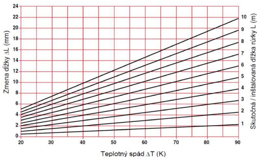
Diagram tepelnej rozťažnosti plastlinikovej rúrky HERZ Pipe Fix
