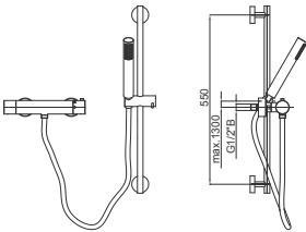
FRESH - ARMATURA ZA PRHO ARMATURA ZA TUŠ SHOWER MIXER-TERMO- STAT
