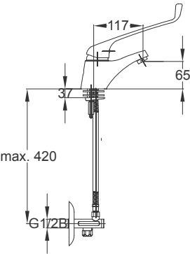
SIMPATY - ARMATURA ZA UMIVALNIK ARMATURA ZA UMIVAONIK BASIN MIXER
