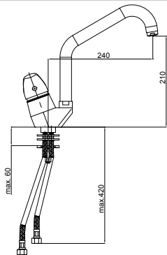
SIMPATY - ARMATURA ZA KUHINJO ARMATURA ZA KUHINJU KITCHEN MIXER
