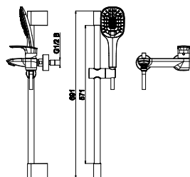
ELITE - ARMATURA ZA KAD ARMATURA ZA KADU BATH/SOWER MIXER
