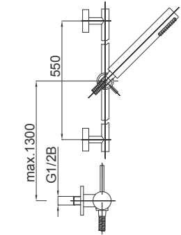
FRESH - ARMATURA ZA PRHO ARMATURA ZA TUŠ SHOWER MIXER
