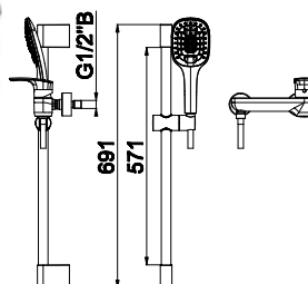
ELITE - ARMATURA ZA PRHO ARMATURA ZA TUŠ SHOWER MIXER
