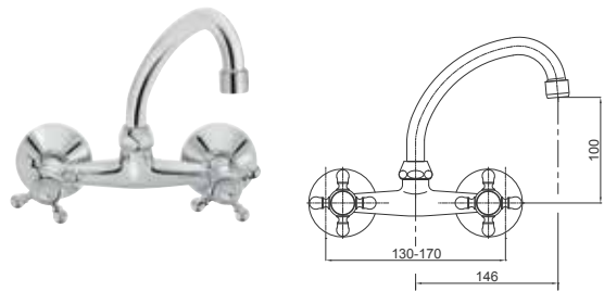
STIL - ARMATURA ZA KUHINJO ARMATURA ZA KUHINJU KITCHEN MIXER
