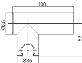
PURE - ZIDNO DRŽALO ZA TUŠ ZIDNI DRŽAČ TUŠA WALL SHOWER HOLDER
