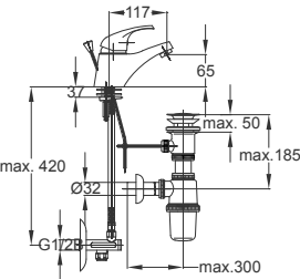
SIMPATY - ARMATURA ZA UMIVALNIK ARMATURA ZA UMIVAONIK BASIN MIXER
