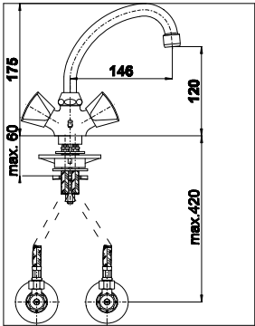
KLASIK - ARMATURA ZA KUHINJO ARMATURA ZA KUHINJU KITCHEN MIXER
