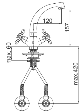
STIL - ARMATURA ZA UMIVALNIK ARMATURA ZA UMIVAONIK BASIN MIXER
