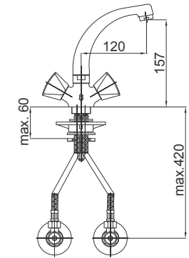
KLASIK - ARMATURA ZA UMIVALNIK ARMATURA ZA UMIVAONIK BASIN MIXER
