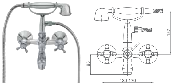
STIL - ARMATURA ZA KAD ARMATURA ZA KADU BATH/SHOWER MIXER
