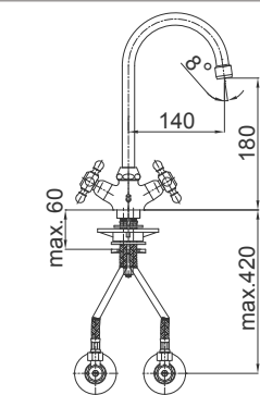
STIL - ARMATURA ZA UMIVALNIK ARMATURA ZA UMIVAONIK BASIN MIXER
